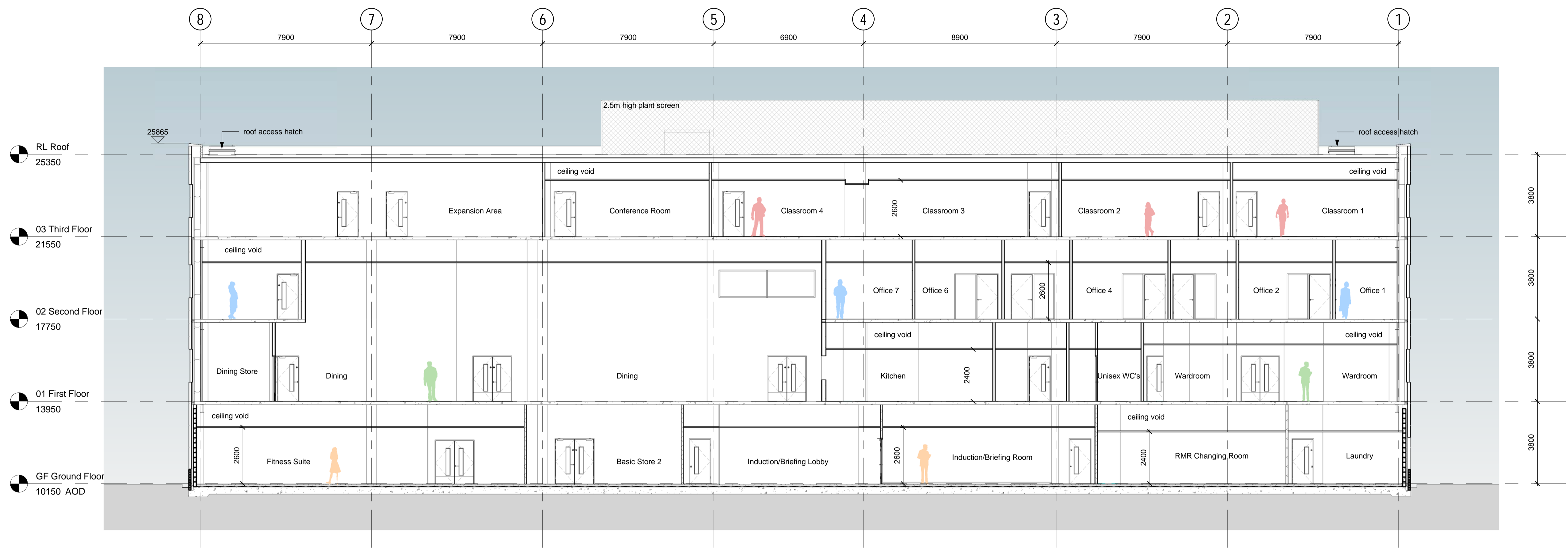
A Section A-A 1 : 100
